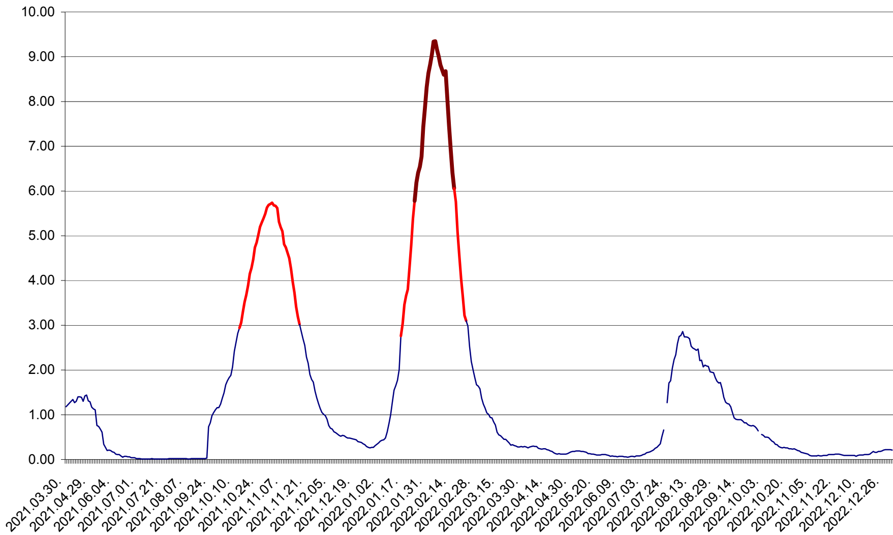
Total - Evolutia incidentei cumulate pe 14 zile la ‰ de locuitori 2021.04.01. - 2022.12.31.
